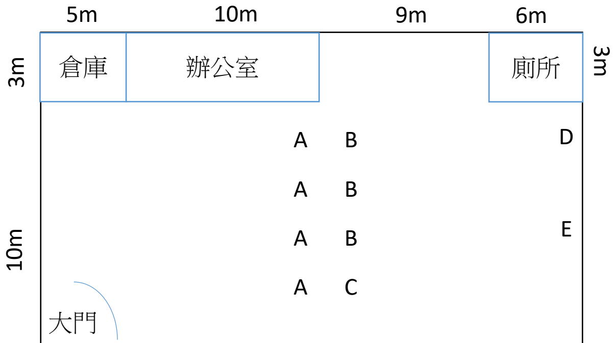
平面圖比例=1/500
